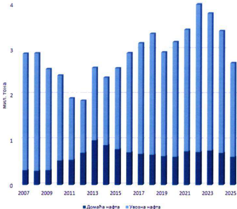
Слика 5-2: Транспортоване количине сирове нафте нафтоводом Транснафта у периоду 2007 – 2025. године
