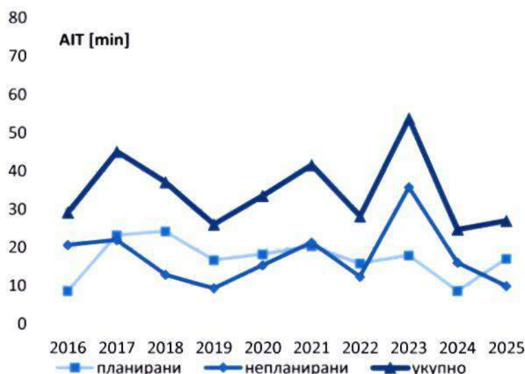
Слика 3-21: Просечно трајање прекида напајања
