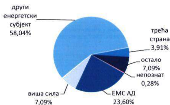
Слика 3-20: Узроци непланираних прекида и њихово учешће у неиспорученој енергији за све кориснике преносног система (укључујући реверзибилне хидроелектране, складишта и пумпно-акумулациона постројења), у 2025. години
