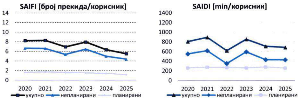
Слика 3-22: SAIFI и SAIDI за период 2020 - 2025. година
