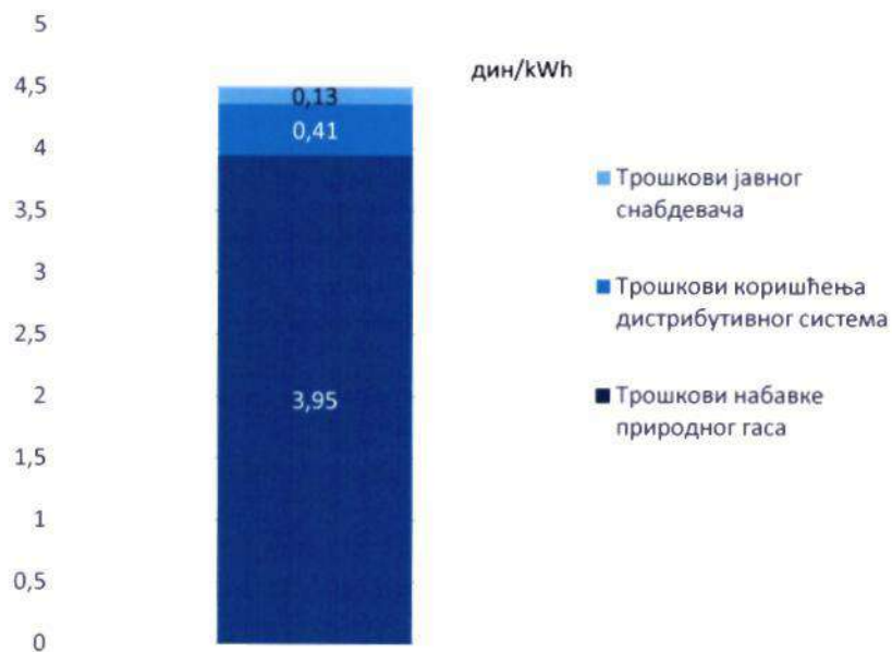
Слика 4-7: Структура просечне одобрене цене природног гаса за јавно снабдевање ЈП Србијасгас на дан 31.12.2025.
