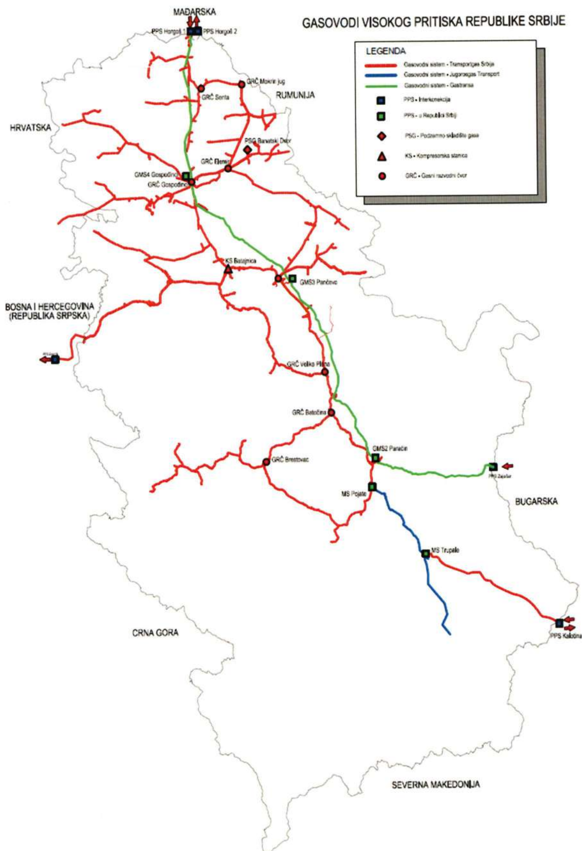
Слика 4-2: Транспортни систем природног гаса Републике Србије
