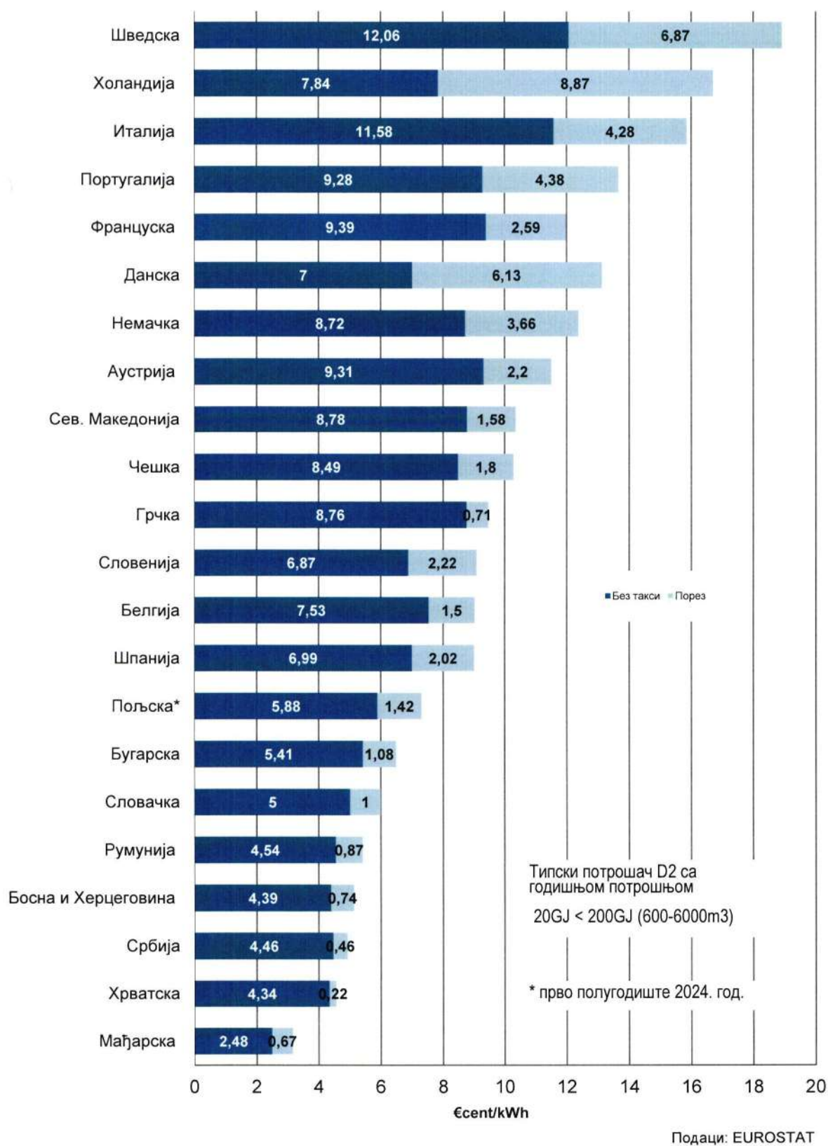
Слика 4-8: Цене природног гаса за домаћинства – друго полугодиште 2024. године
