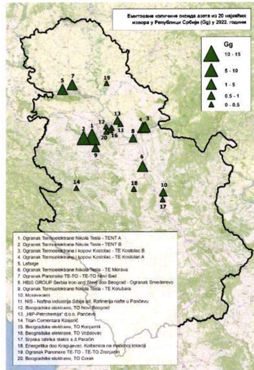
Слика 3.2.2. 20 најзначајнијих извора азотних оксида у Републици Србији
