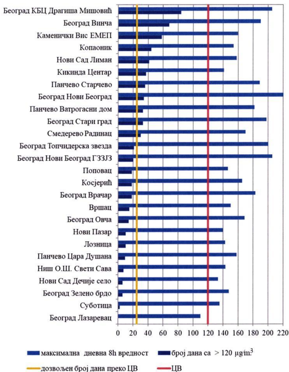
Слика 3.1.21. Упоредни приказ максималних дневних осмосатних концентрација \text{O}_3 ( \mu\text{g}/\text{m}^3 ) и броја дана са прекорачењем ЦВ у 2022. години
