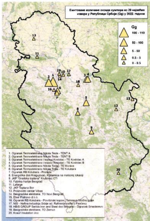
Слика 3.2.1. 20 најзначајнијих извора сумпор диоксида у Републици Србији
