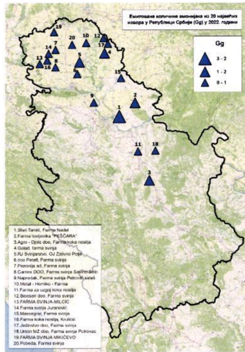
Слика 3.2.4. 20 најзначајнијих извора амонијака у Републици Србији
