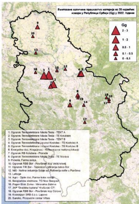
Слика 3.2.3. 20 најзначајнијих извора прашкастих материја у Републици Србији
