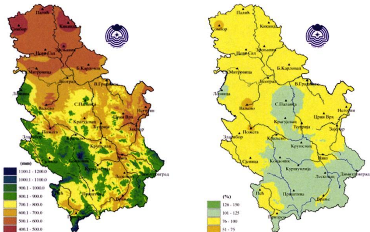
Слика 3.3.20. Распореда количина падавина (mm) на подручју Републике Србије у 2022. години (лево) и одступања годишње количине падавина у процентима од нормале 1991-2020. (десно)
