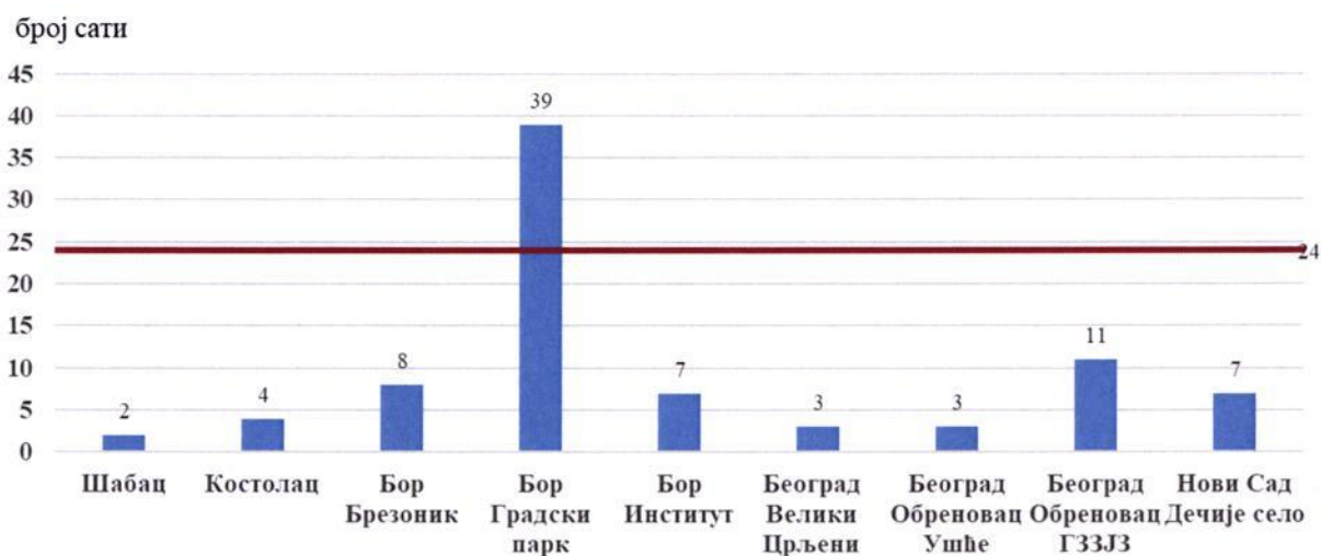
Слика 3.1.8. Мерна места у Републици Србији током 2022. године на којима је регистровано прекорачење сатне граничне вредности сумпор диоксида
