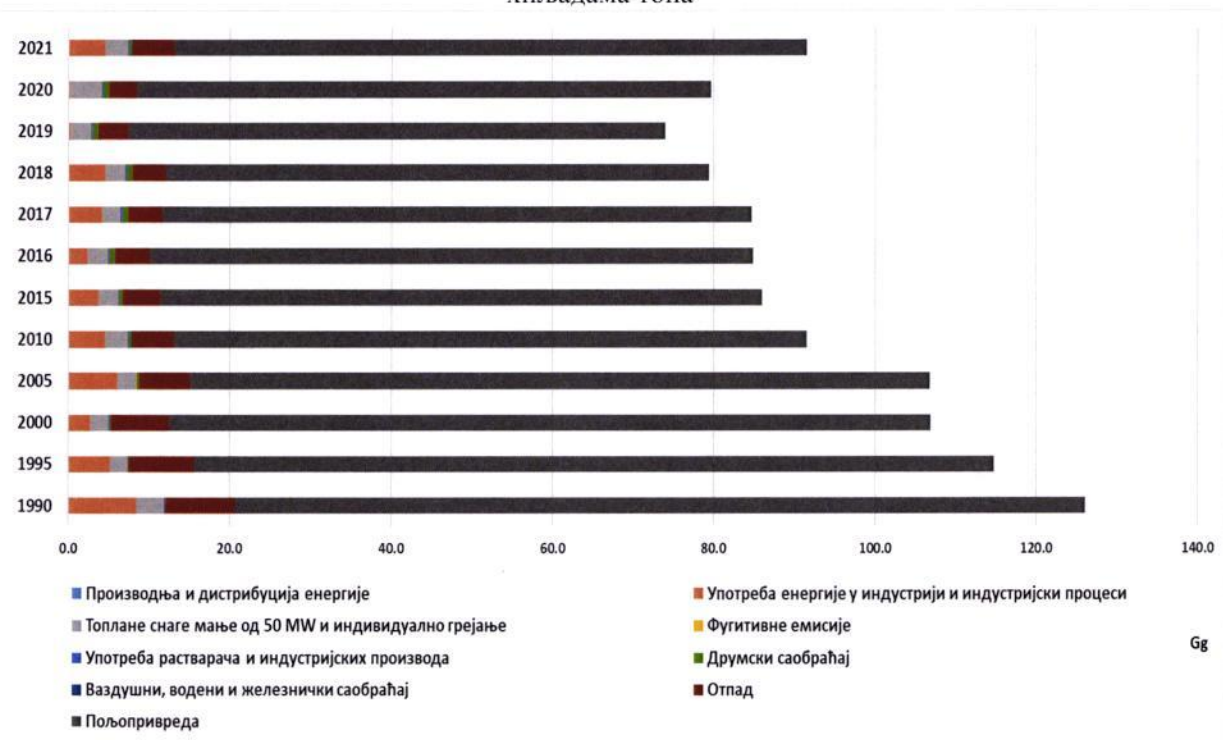
Слика 3.2.8. Емисије амонијака по секторима у периоду 1990-2021. године изражена у хиљадама тона
