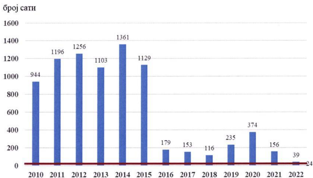
Слика 3.1.9. Број сати током године када је концентрација сумпор диоксида прекорачила граничну вредност ( 350 \mu\text{g}/\text{m}^3 ) на станици Бор Градски парк у периоду 2010-2022. године (дозвољено је 24 сата са прекорачењем током календарске године)
