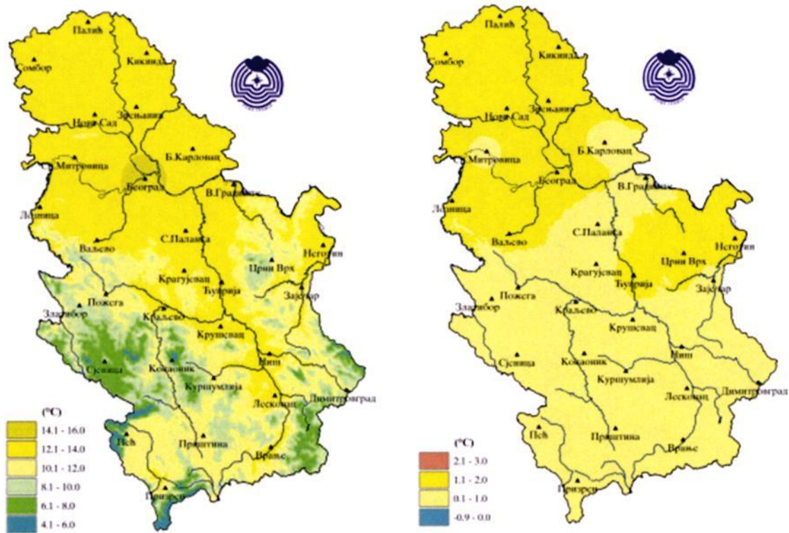
Слика 3.3.21. Распдела годишњих вредности температуре (°C) на подручју Републике Србије у 2022. години (лево) и одступања средње годишње температуре у (°C) од нормале 1991-2020. (десно)
